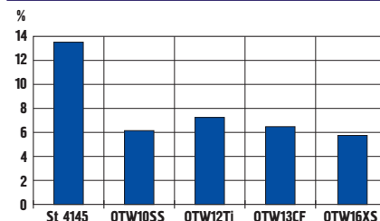
ИЗНОС ОБСАДНОЙ ТРУБЫ В %, ТЕСТ МОНР
